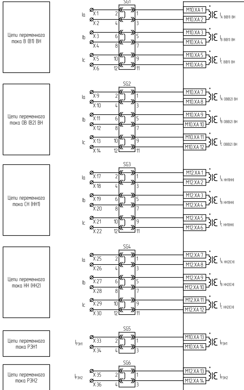
Цепи переменного тока А1
