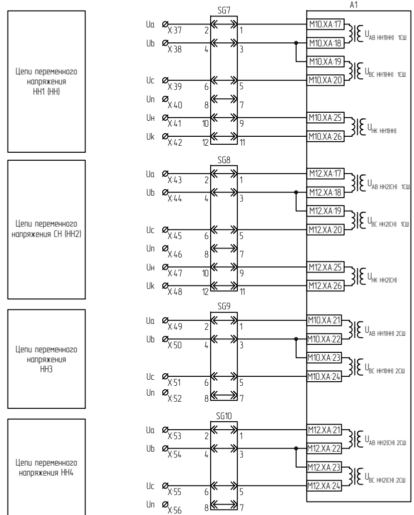
Цепи переменного и напряжения А1
